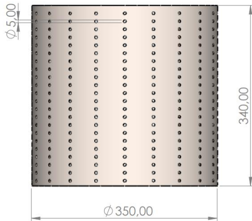
Gambar 6. Desain tabung pengupas kulit kentang (ukuran dalam mm)
