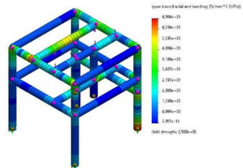
Gambar 3. Hasil simulasi von misses stress
