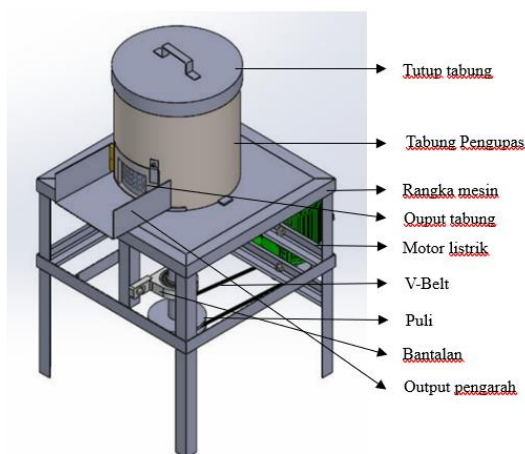
Gambar 2. Desain mesin pengupas kulit kentang
