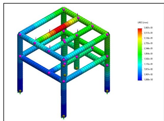
Gambar 4. Hasil simulasi displacement
